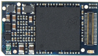
OMAP35x Torpedo™ SOM
